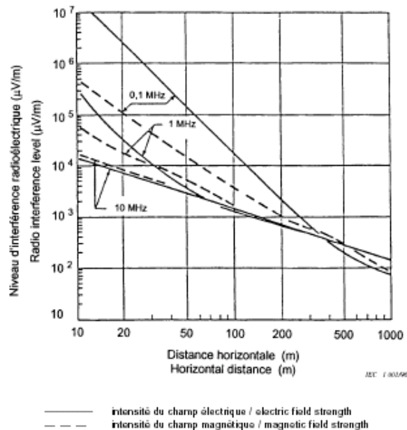
Figure 17 – Atténuation du niveau perturbateur en fonction de la distance sur un plan horizontal pour différentes fréquences (Valeurs calculés de la radiation libre provoquée par un dipôle électrique vertical; voir référence [77])
